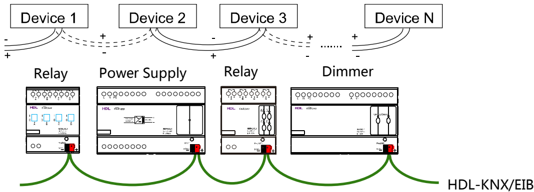
KNX/EIB Wiring Diagram:
