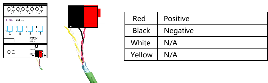
KNX/EIB Wiring Diagram:
